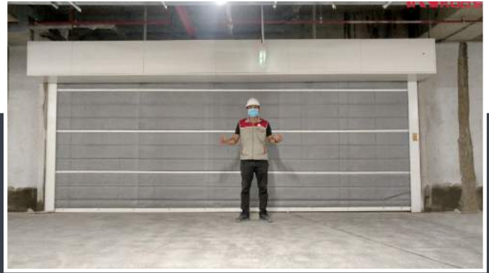
MÀN CUỐN NGẮN CHÁY MỘT THÂN GHCL E160
